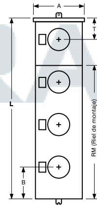
Sección derivada
