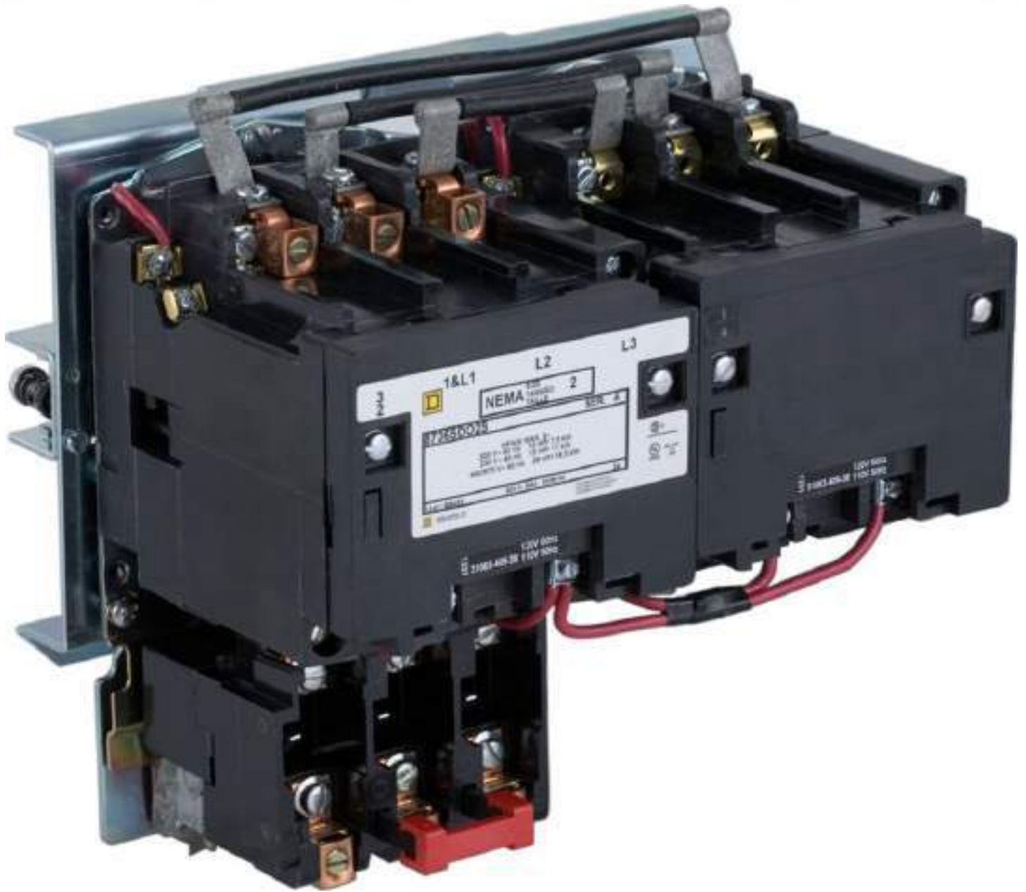
Arranadores magnéticos reversibles Clase 8736S
