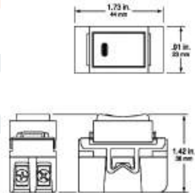
Rocker Switch (SERPRWS)
