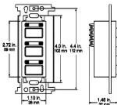
Botón pulsador (SERPWS)
