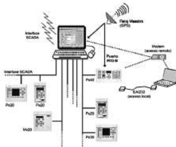
Un sistema de control de subestación típico
